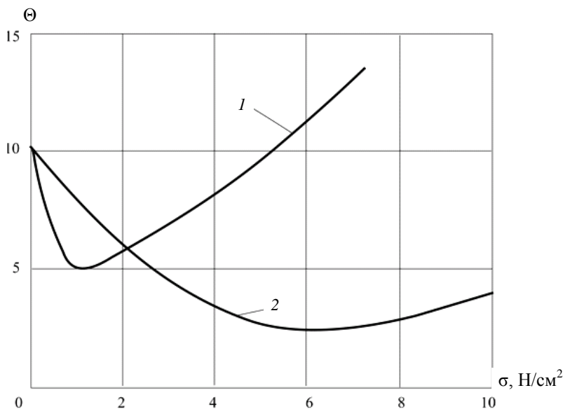
Рис. 3.5. Зависимость \Theta = f(\sigma) для поролона и губчатой резины: 1 – поролон ( \rho = 0,033 \text{ г/см}^3 ); 2 – губчатая резина ( \rho = 0,127 \text{ г/см}^3 )
