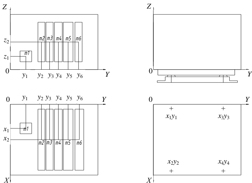
Рис. 3.2. Схема расположения амортизаторов на блоке РЭС
